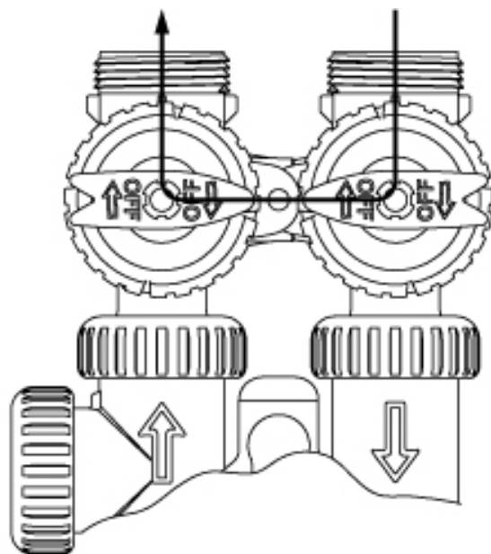
Рисунок 4 Положение Выключен
